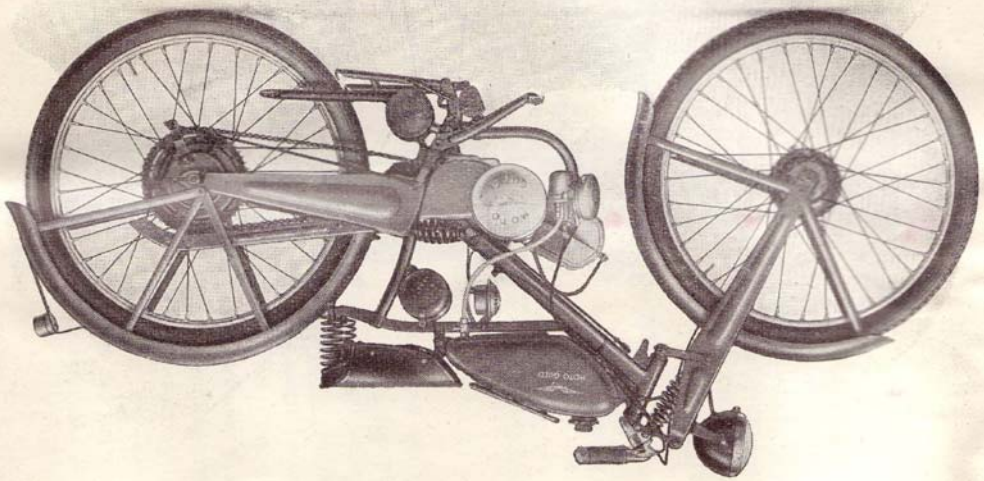
Fig. 2 - Motoleggera (lato volante magnetico)
